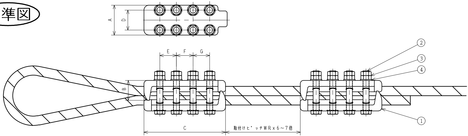
寸法表
